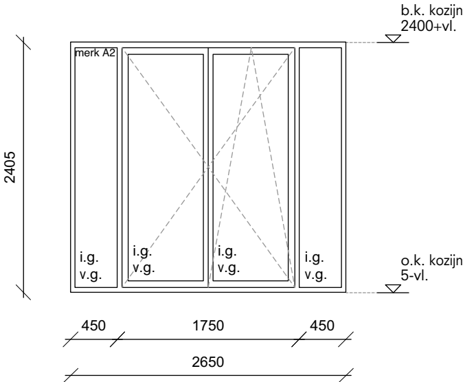
Merk A2
